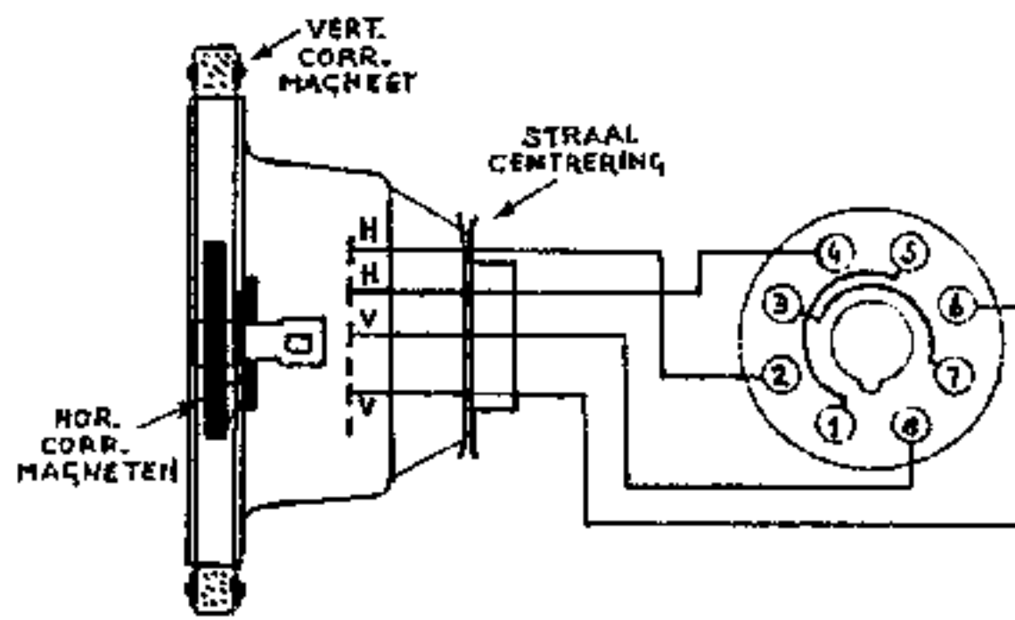
DEFLECTIE JUK DEFLECTION YOKE ABLENKEINHEIT AT 1031 So 057 882
