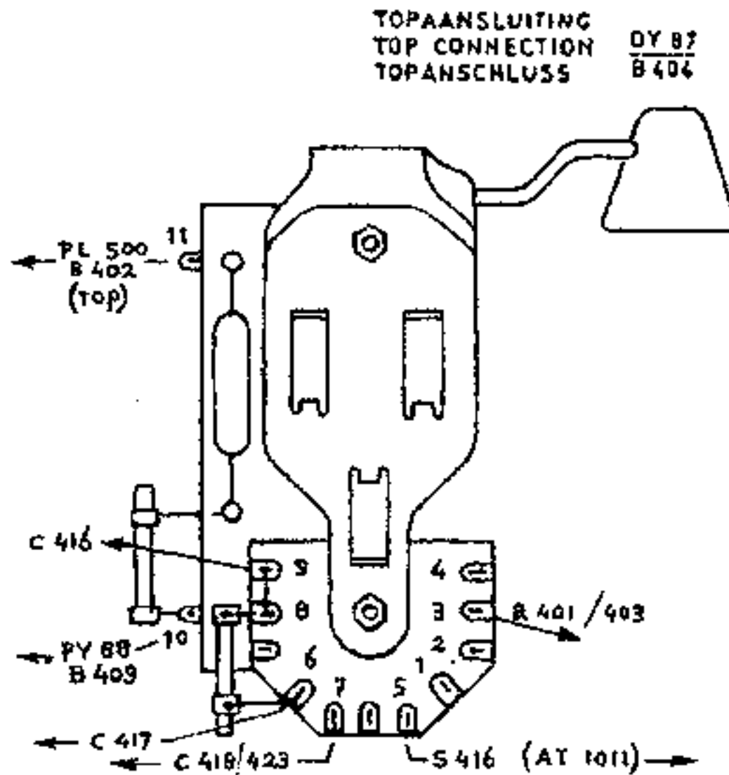
LIJNUITGANGS TRAFU LINE OUTPUT TRANSF. ZEILENAUSG. ÜBERTRAGER AT 2023 So 051 709
